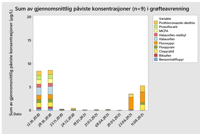
Figur 7.2 Sum av gjennomsnittlig målte konsentrasjoner av plantevernmidler ( \mu\text{g/L} ) i grøfteavrenning fra alle 9 forsøksruter pr prøvetaksdato.
