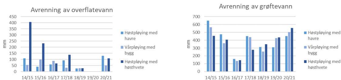
Figur 01. Avrenning på overflaten og gjennom drenggrøftene for 2014/2015-2020/2021 i gjennomsnitt for hver behandling.
