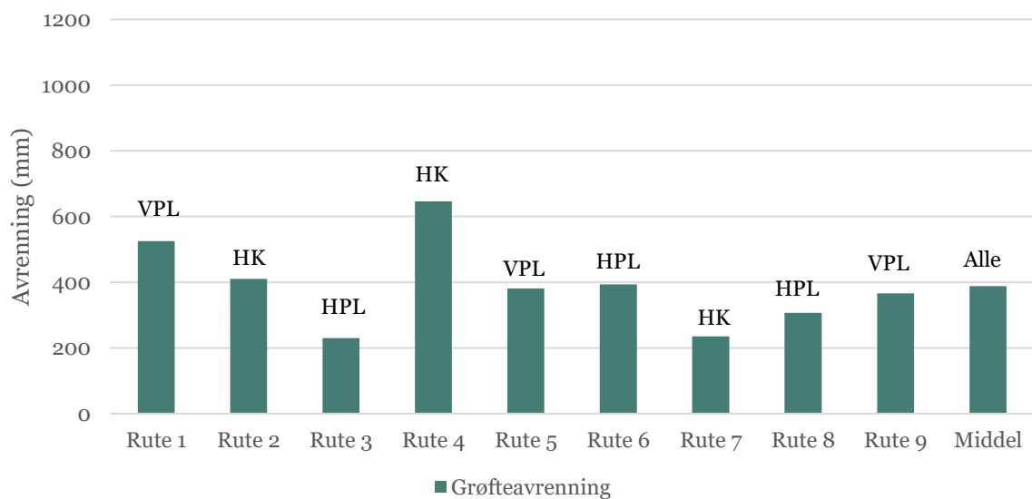
Figur 5.6. Grøfteavrenning (mm) fra rute 1-9 i forsøksperioden 1.9.2019 til 1.9.2020. HK = høstkorn med høstpløying, HPL = høstpløying, og VPL = vårpløying.
