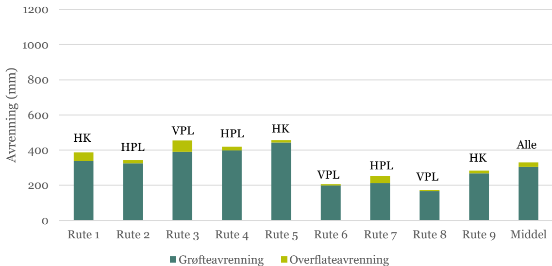
Figur 5.5. Overflate- og grøfteavrenning (mm) fra rute 1-9 i forsøksperioden 1.9.2018 til 1.9.2019. HK = høstkorn med høstpløying, HPL = høstpløying, og VPL = vårpløying.
